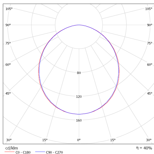
OPAL 2x28W
