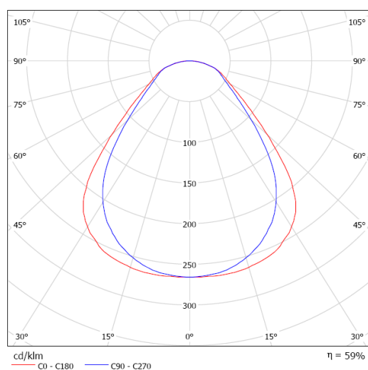
PRISMA 4X24W
