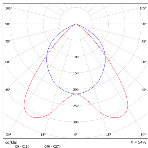
PAR 2X36W
