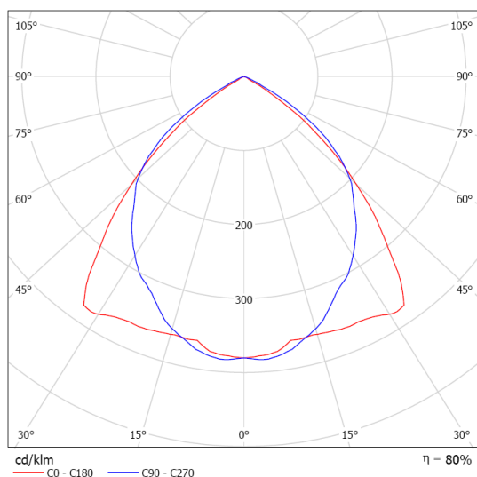
4x14W
