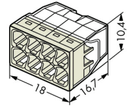
2273-208 8-conductor
